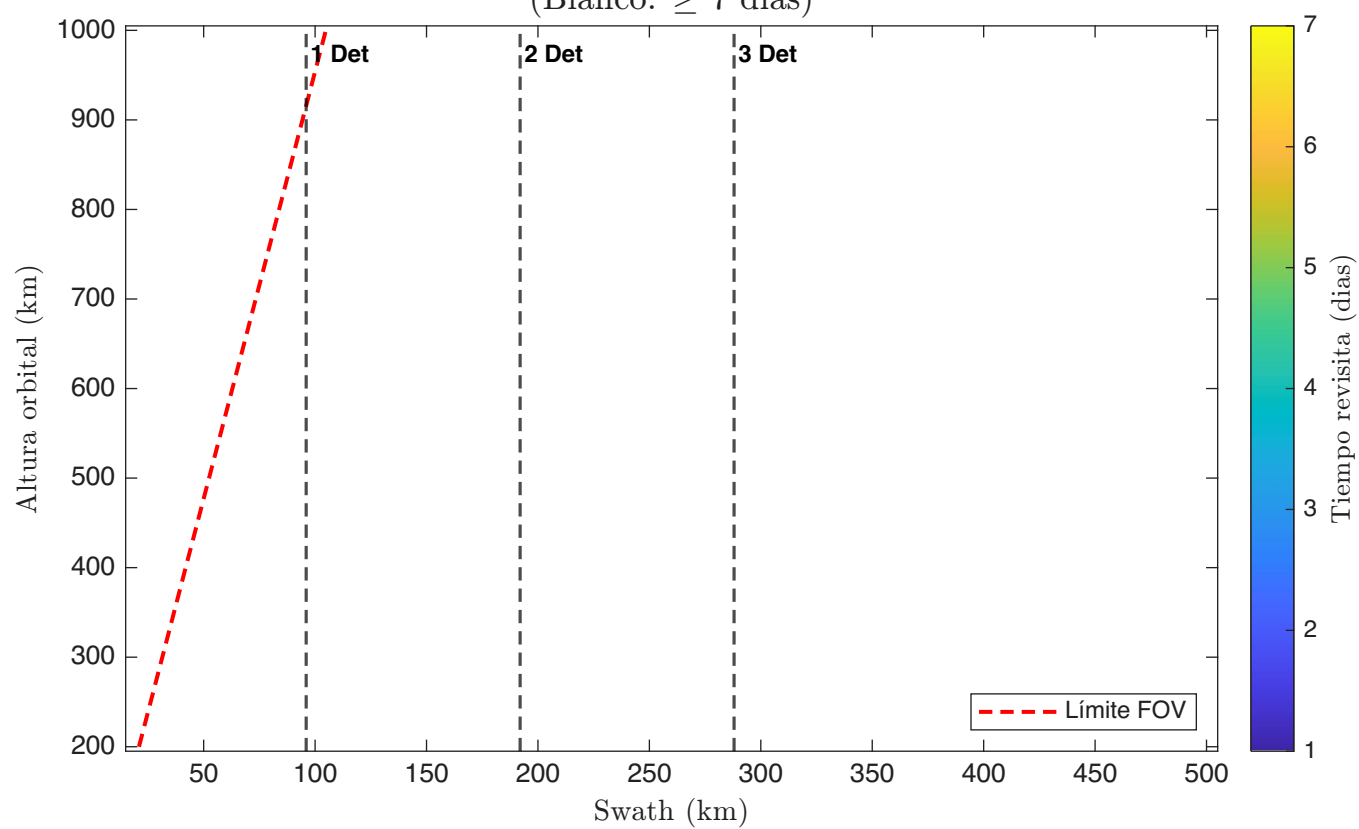
Tiempo Revisita - 1 Satelite(s); 2 Telescopio(s): Korsch; Detector 1 (Blanco: \geq 7 dias)
